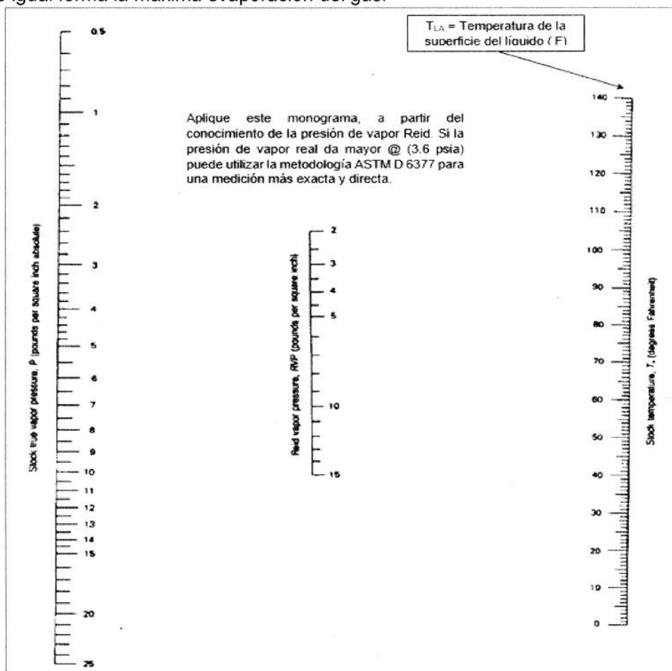
Figura. 7.1-13a Nomograma para cálculo de la presión de vapor real. Presión de vapor real de crudos con una presión de vapor Reid de 2 a 15 libras por pulgada cuadrada. Fuente: Norma API greenhouse Technical compilation.
